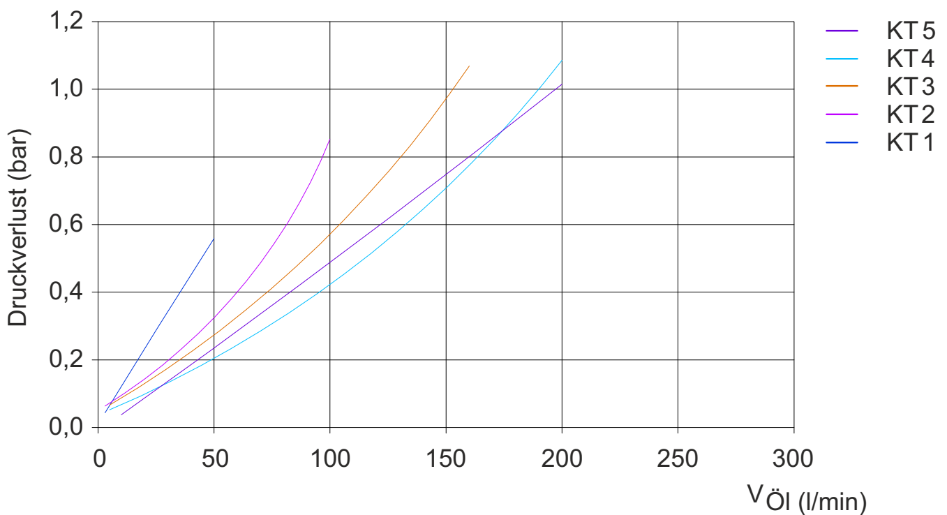
Druckverlustrdiagramm
