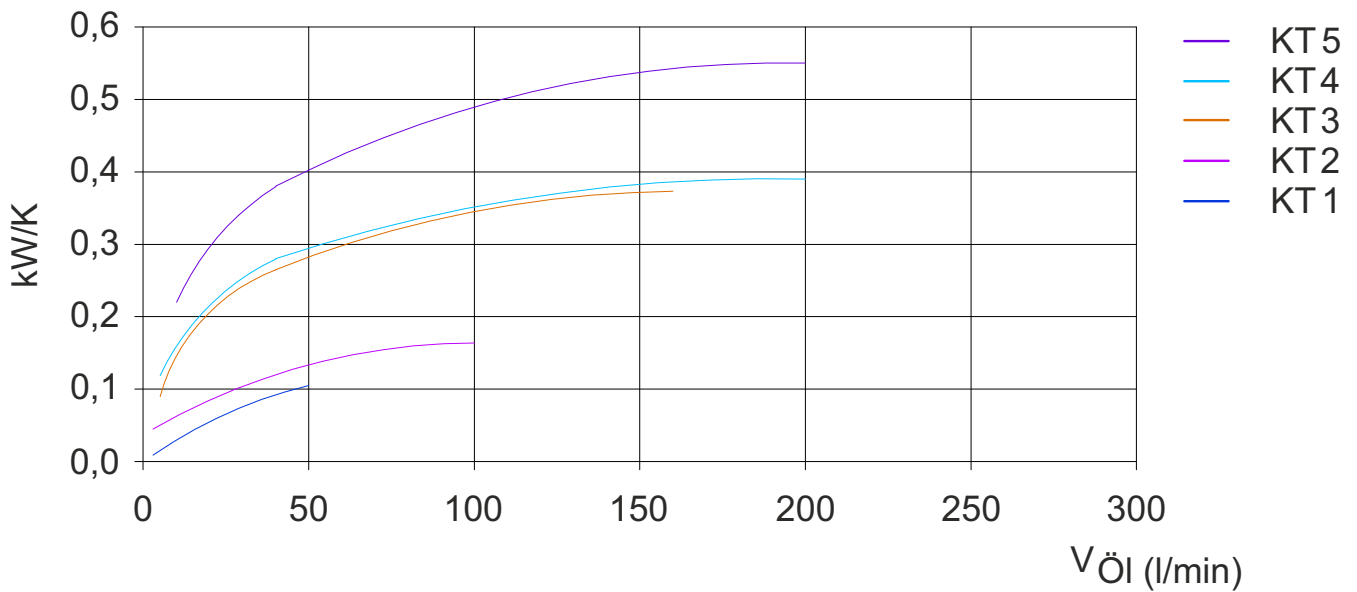
Leistungsdiagramm
