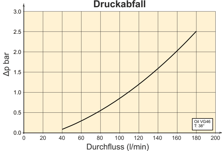
Druckabfall
