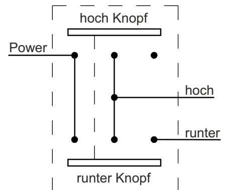
Anschlussdiagramm
