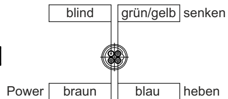
Anschlussdiagramm
