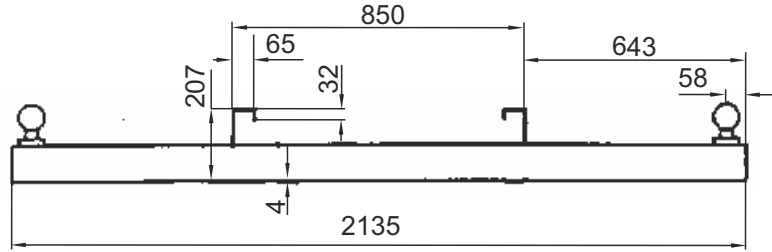
Schnitt - S -
