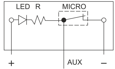
elektr. Anschlussplan
