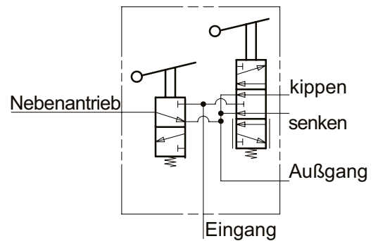
pneum. Anschlussplan
