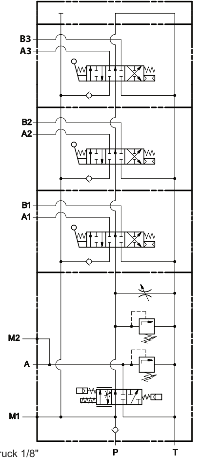
P Druckeingang Pumpe 1"
