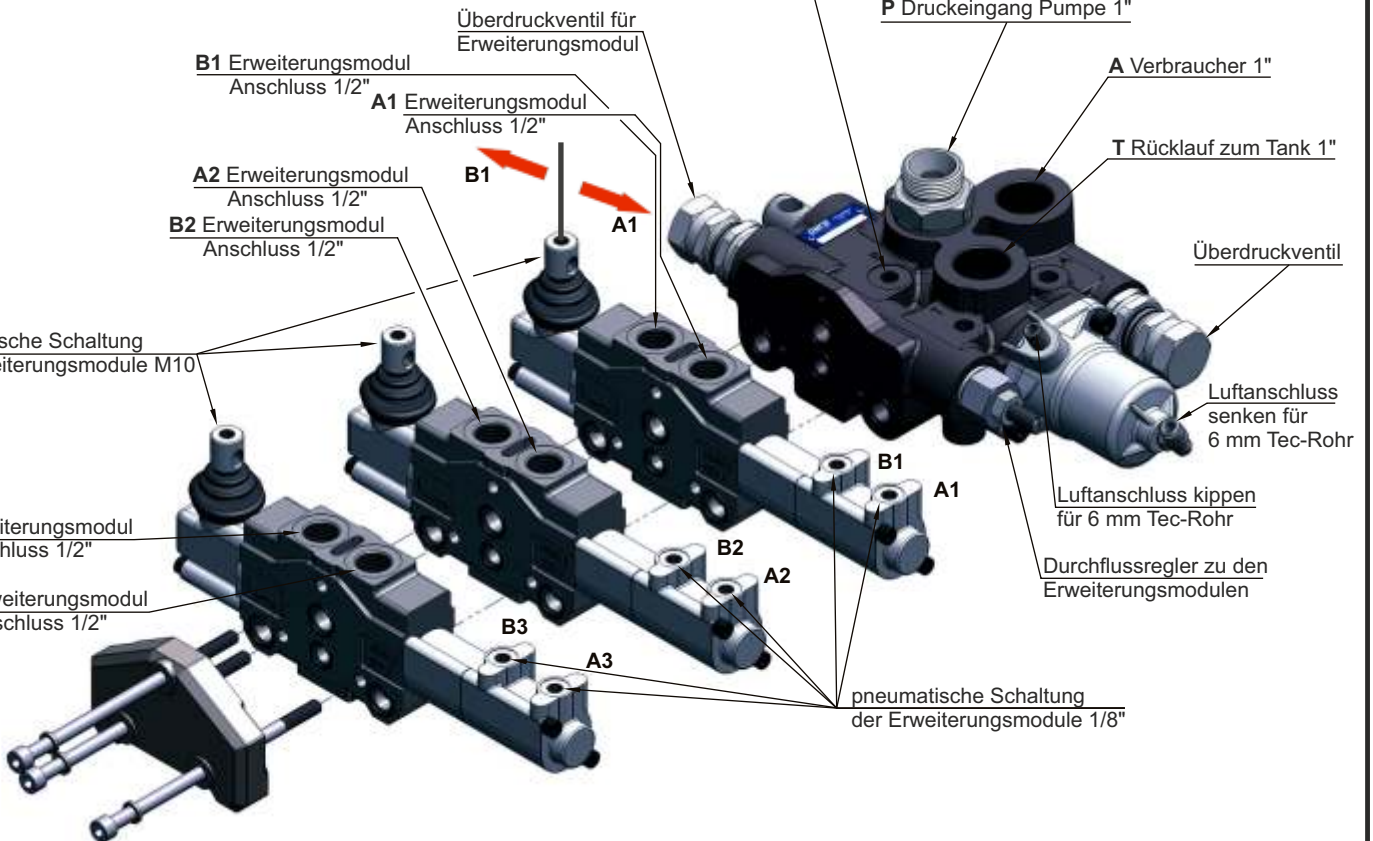
P Druckeingang Pumpe 1"
